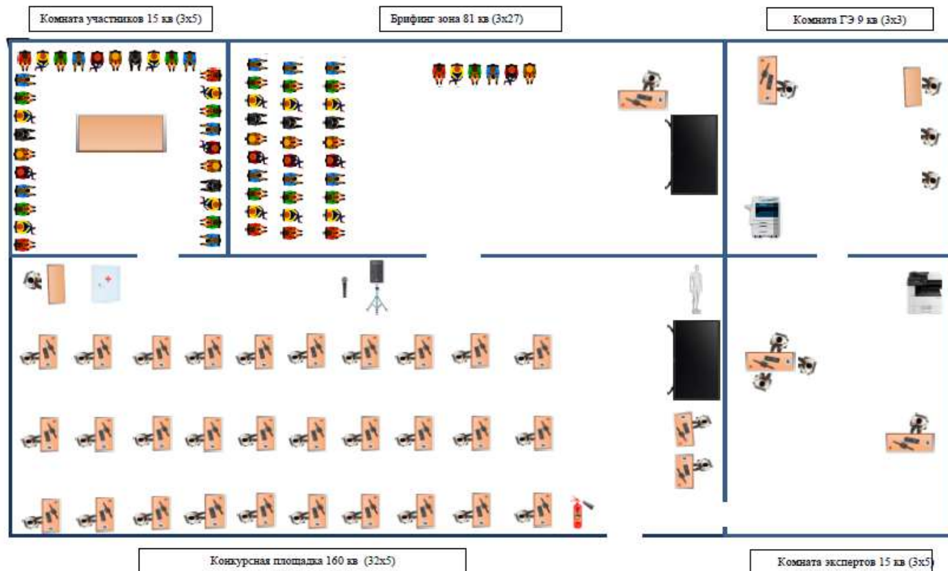
Рисунок VII.1 - План застройки площадки центра проведения демонстрационного экзамена
