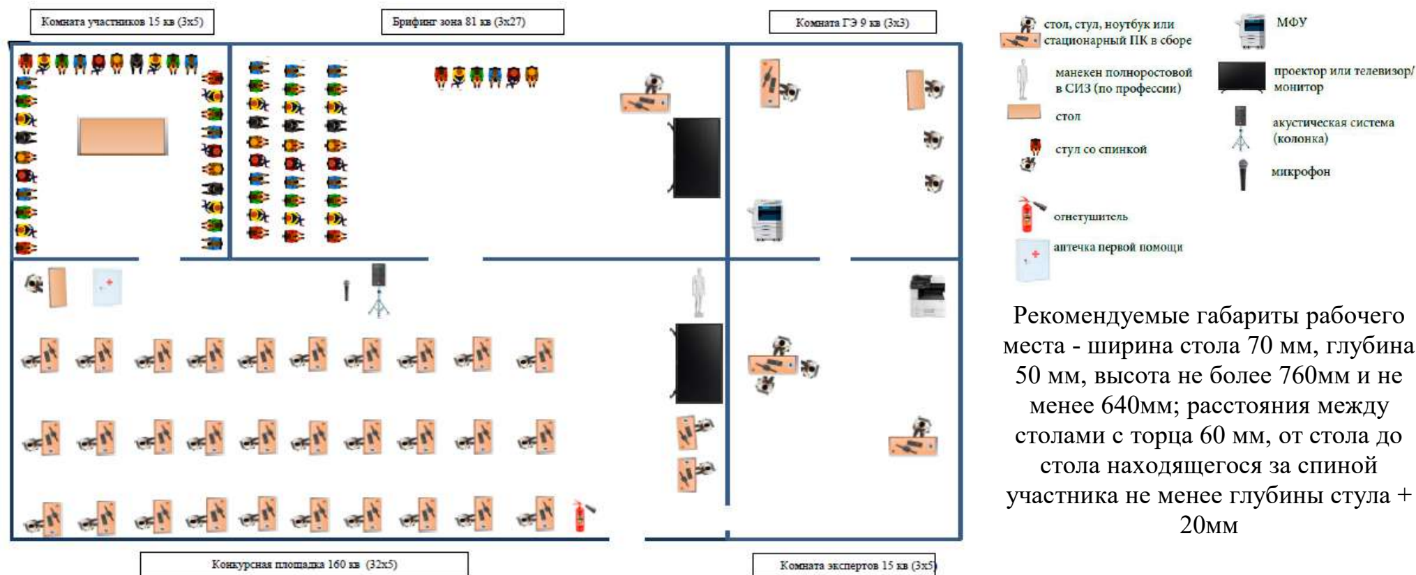
Рисунок V.1 - План застройки площадки центра проведения демонстрационного экзамена
