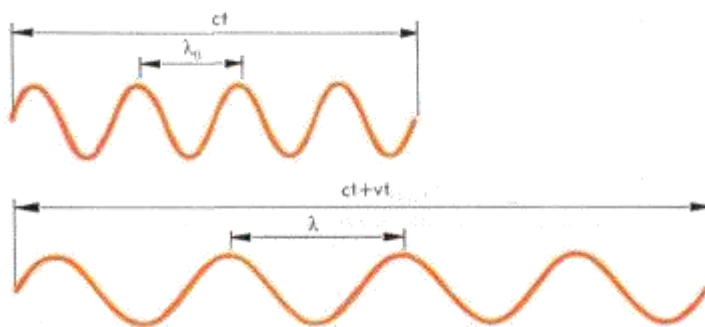
К объяснению эффекта Доплера.
